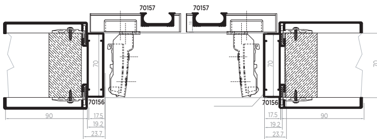
SECCIÓN LONGITUDINAL 2 HOJAS SECTION LONGITUDINALE 2 OUVRANTS
